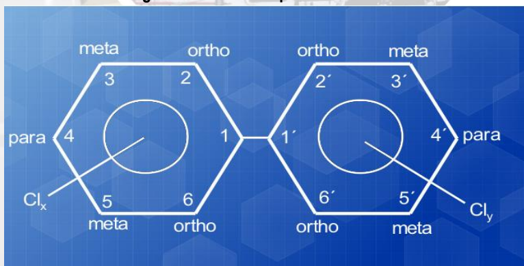
Figura 1. Estructura química de los PCB
