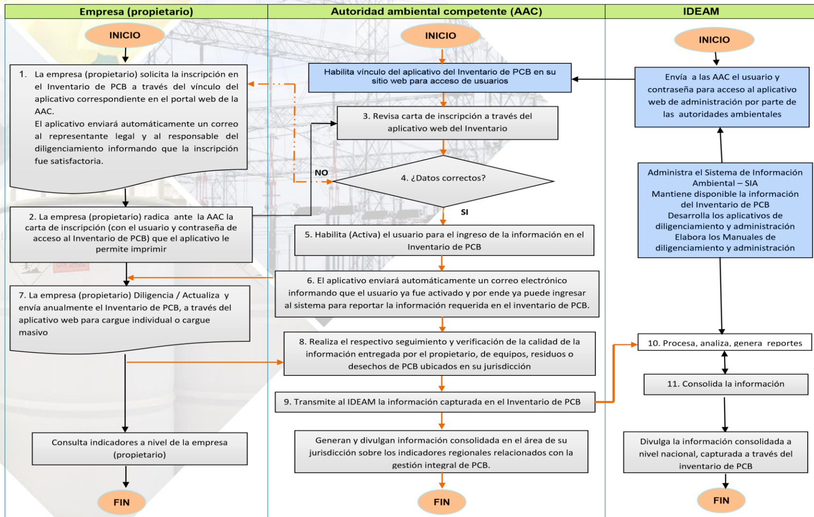
Figura 4. Diagrama de flujo del proceso de implementación del Inventario Nacional de PCB.
