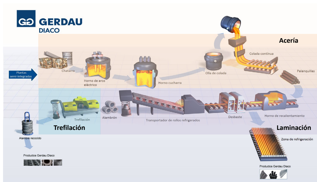
Figura 11. Ejemplo de proceso siderúrgico en planta semiintegrada
